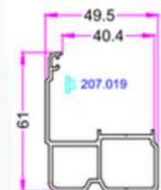
BATTEMENT (POUR PORTILLON)
